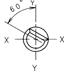
軸は、反時計方向に 回し切った状態を示す SHAFT SHOWN IN FULL C.C.W POSITION.
