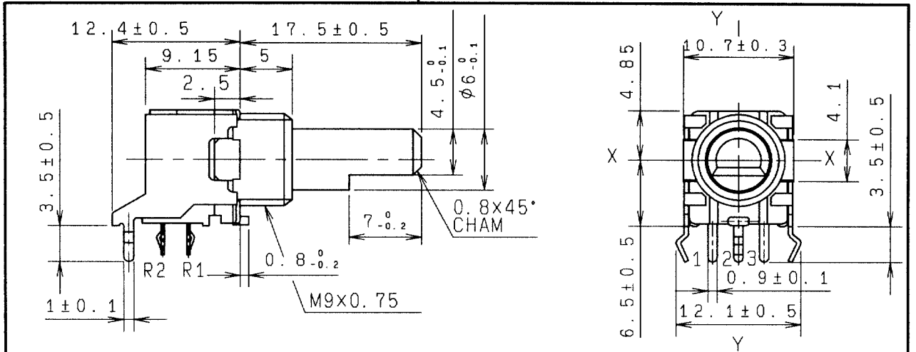
軸はセンタークリック位置を示す SHAFT SHOWN IN CENTER CLICK POSITION
